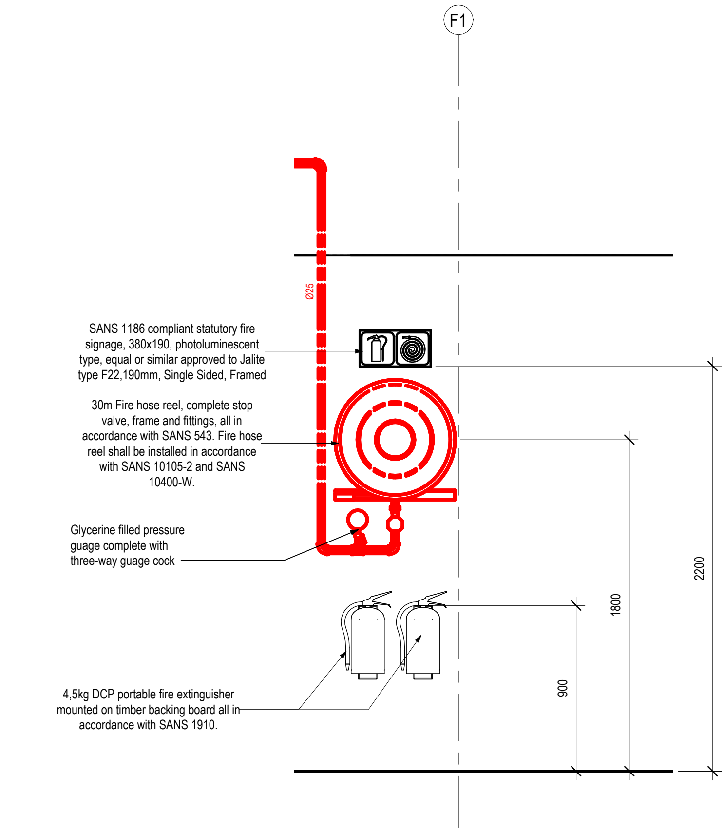
2 Elevation 1 - a 1 : 20
